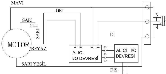
ÇİFT HIZ INFRARED UZAKTAN KUMANDA TEL BAĞLANTI ŞEMASI
